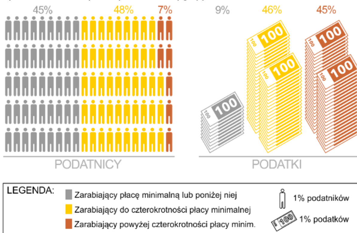
Rysunek 36. Podatnicy PIT w podziale na trzy grupy dochodowości
