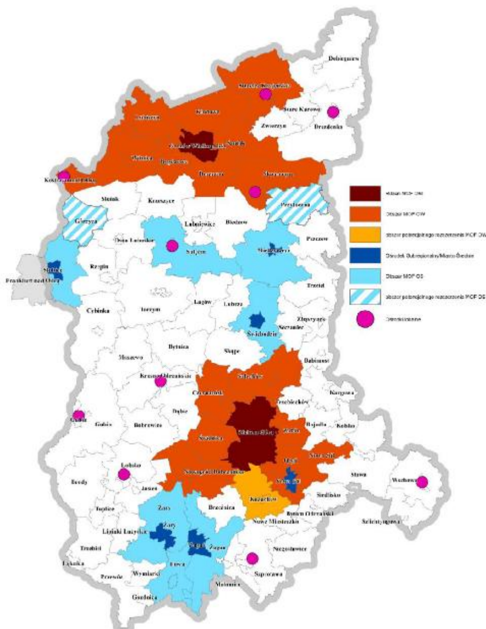
Rysunek 1. Delimitacja ŚMMOF w strategii wojewódzkiej
