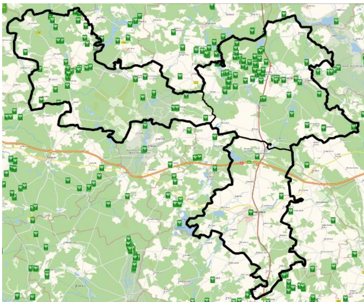
Rysunek 24. Pomniki przyrody na obszarze Partnerstwabszarze Partnerstwa
