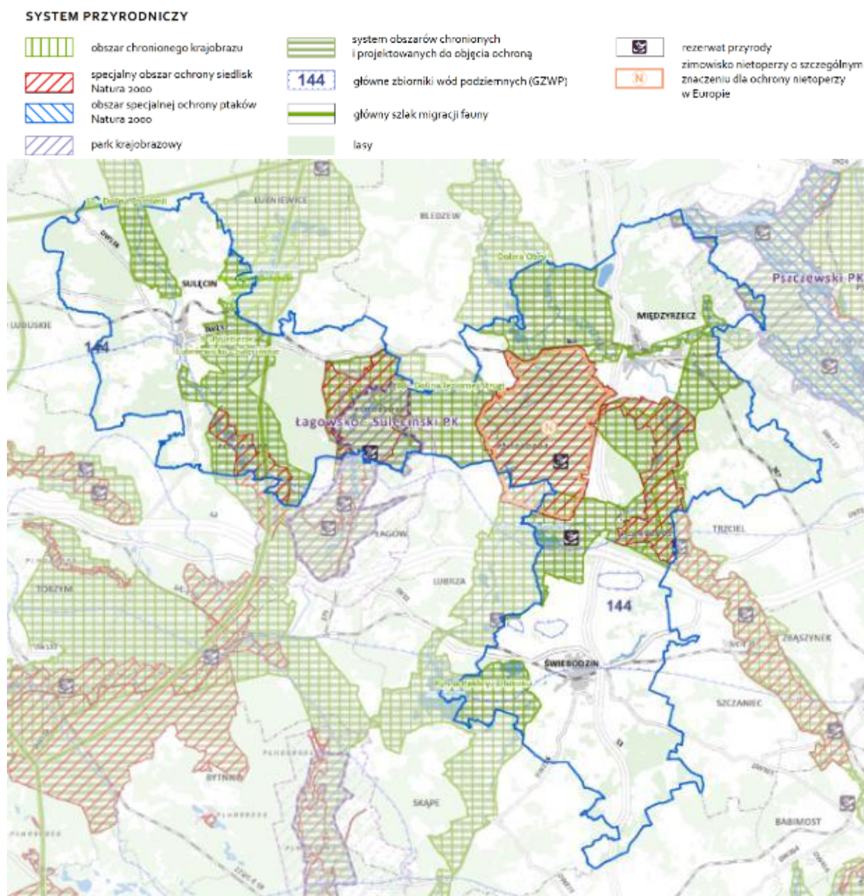
Rysunek 57. Partnerstwo Świebodzińsko-Międzyrzecki MOF – Ochrona i kształtowanie środowiska, system powiązań przyrodniczych
