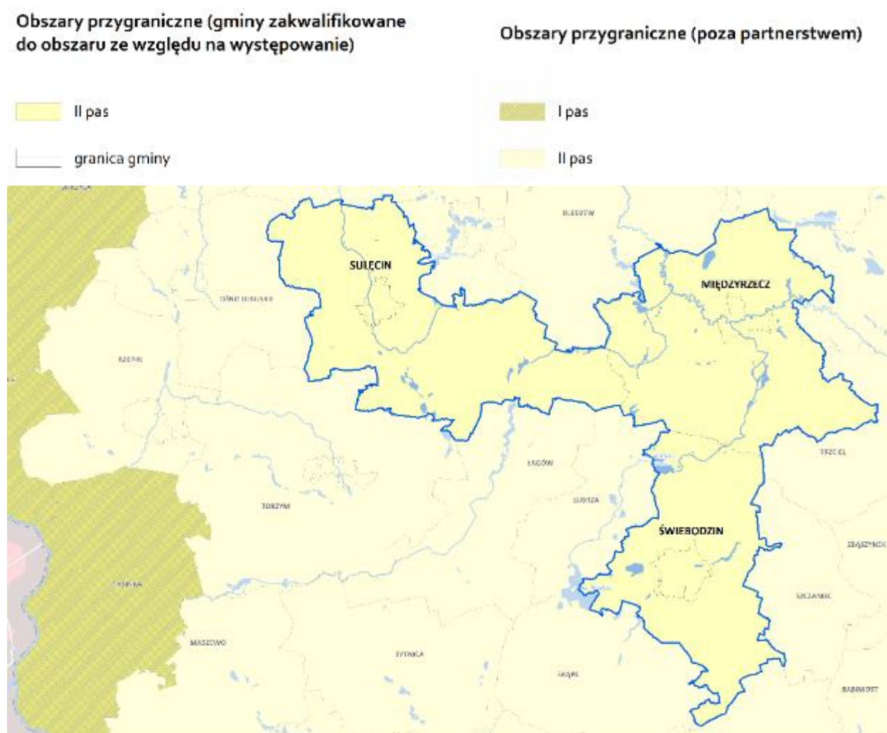
Rysunek 65. OSI - Obszary przygraniczne określone w SRWL 2030
